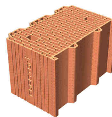
Blocco rettificato POROTON® denominato "P600 IT38 SS ECO DRY-PLAN", dimensioni nominali 230 x 380 x 240 mm
