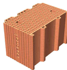
Blocco POROTON® denominato "P600 IT38 SS", dimensioni nominali 230 x 380 x 240 mm
